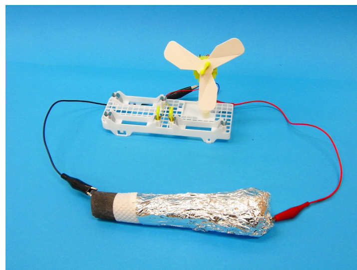
(配線例)
